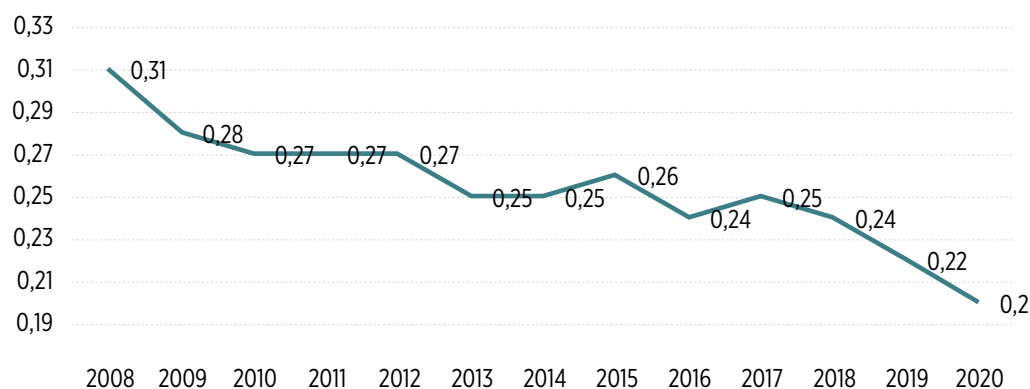
GRÁFICO 18. EMISIONES DE CO 2 DE LAS UNIDADES RESIDENTES (KG CO 2 EQUIVALENTE/ EUROS) POR PIB
