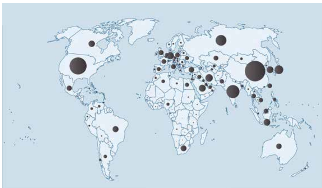
GRÁFICO 3: EMISIONES DE CO 2 POR PAÍSES. 2020
