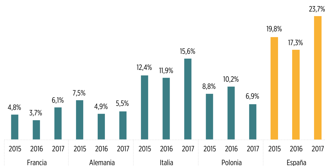
GRÁFICO 6. ÍNDICE DE EXPLOTACIÓN WEI+ POR AÑO Y PAÍS (UNIDADES: % DE AGUA USADA)
